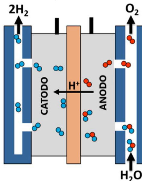
Figura 4. Proceso de electrólisis con electrolizador PEM
