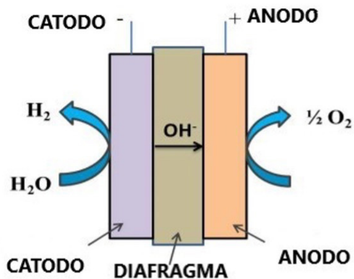
Figura 5. Electrolizador alcalino
